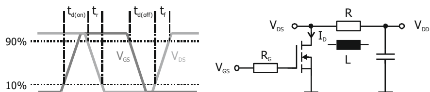
Fig. 1 Test circuit for switching times (R) and avalanche energy (L) ("rise" and "fall" refer to I_D ) Testaufbau für Schaltzeiten (R) und Avalanche-Energie (L) ("rise" und "fall" beziehen sich auf I_D )
