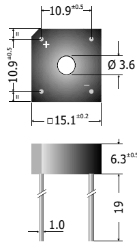
Dimensions - Maße [mm]
