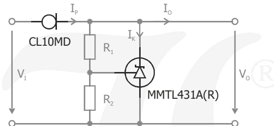
Fig. 3 Spannungsversorgung mit geringem Bauteilbedarf für \mu Controller und andere Schaltungen mit niedrigem Eingangsstrom
