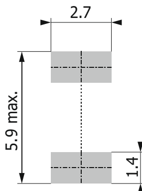
SMB DO-214 AA
