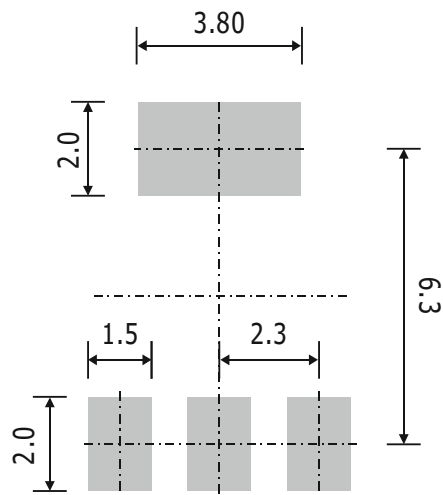
SOT-223
