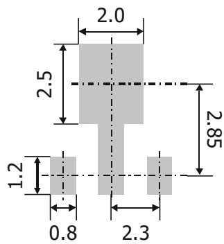
SOT-89
