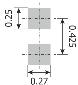
0201 (0603)
