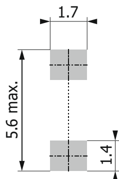
SMA DO-214 AC
