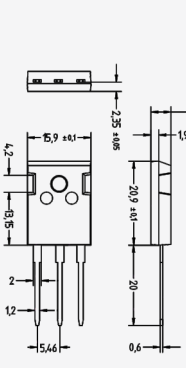
TO-247-3L
