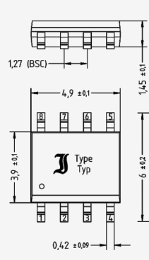
SO-DIL
