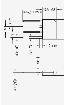
DB
