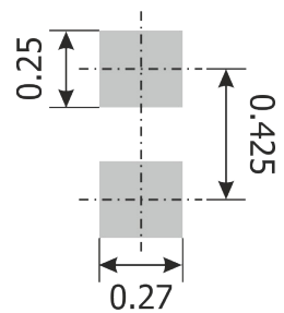
0201 (0603)
