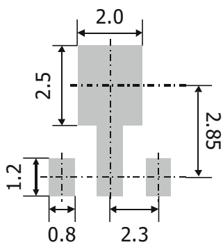
SOT-89
